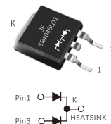
TO-263 SR4045LD1
