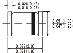
MicroMelf
