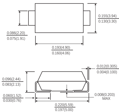
SMB(DO-214AA)
