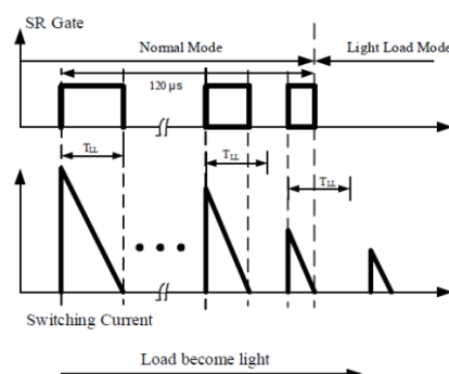
图 5 进入轻载模式示意图
